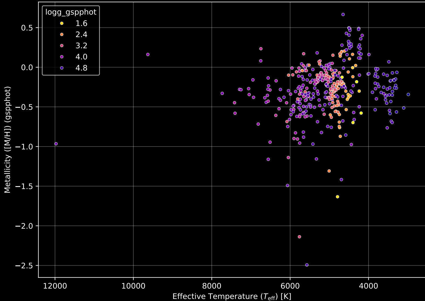
APOGEE DR17 Field: [150+30] Stellar Population Parameters (n= 404)
